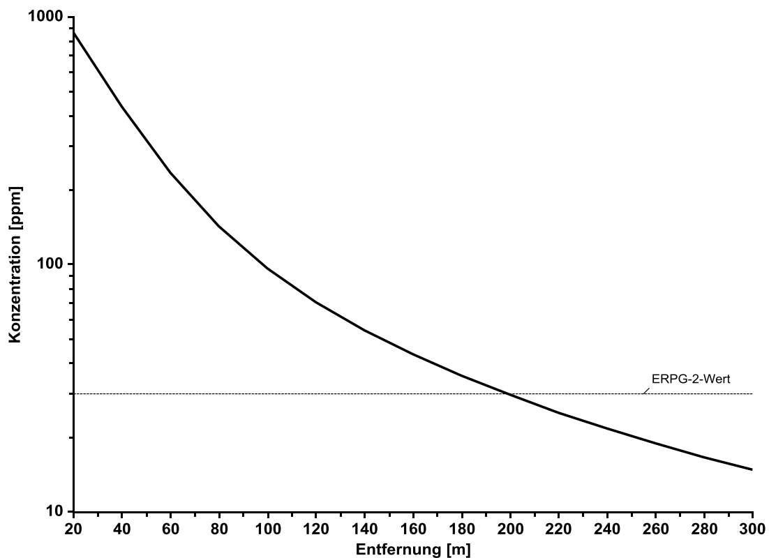
Bild 1: Schwefelwasserstoff-Konzentration bei der Freisetzung von 18,6 kg/s Biogas
